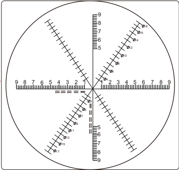
水平和垂直方向为长度刻线，分度值为0.2mm； 两条斜线为直径刻线，分度值为1mm (当使用1X物镜时)
